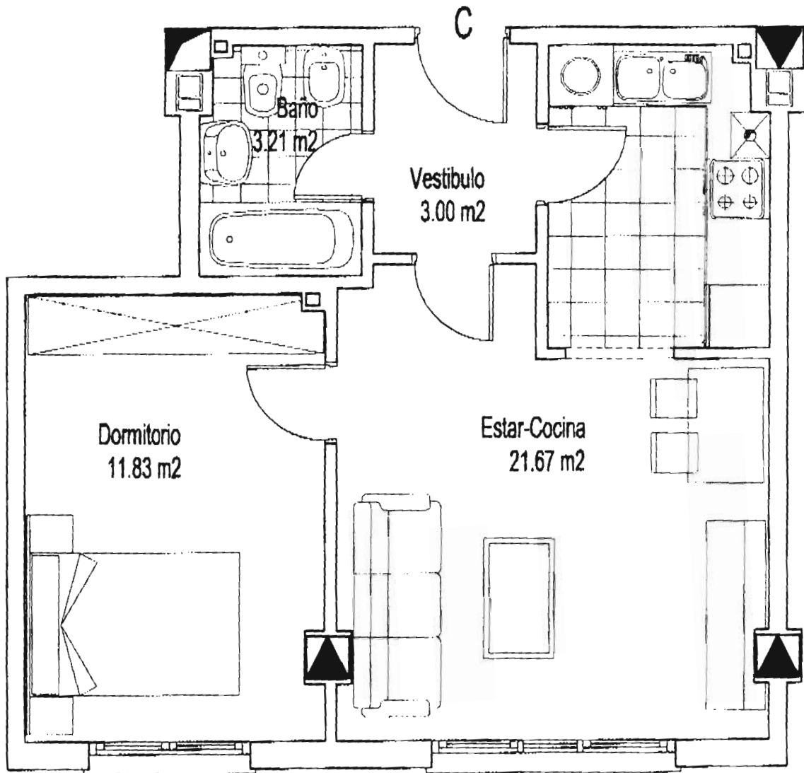
ORIENTACION OESTE VIVIENDA C PLANTA PRIMERA Y SEGUNDA - MUEBLES BLOQUE 3 ESCALA 1/50
