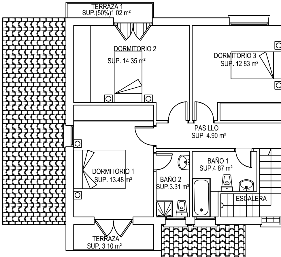
PLANTA PRIMERA
