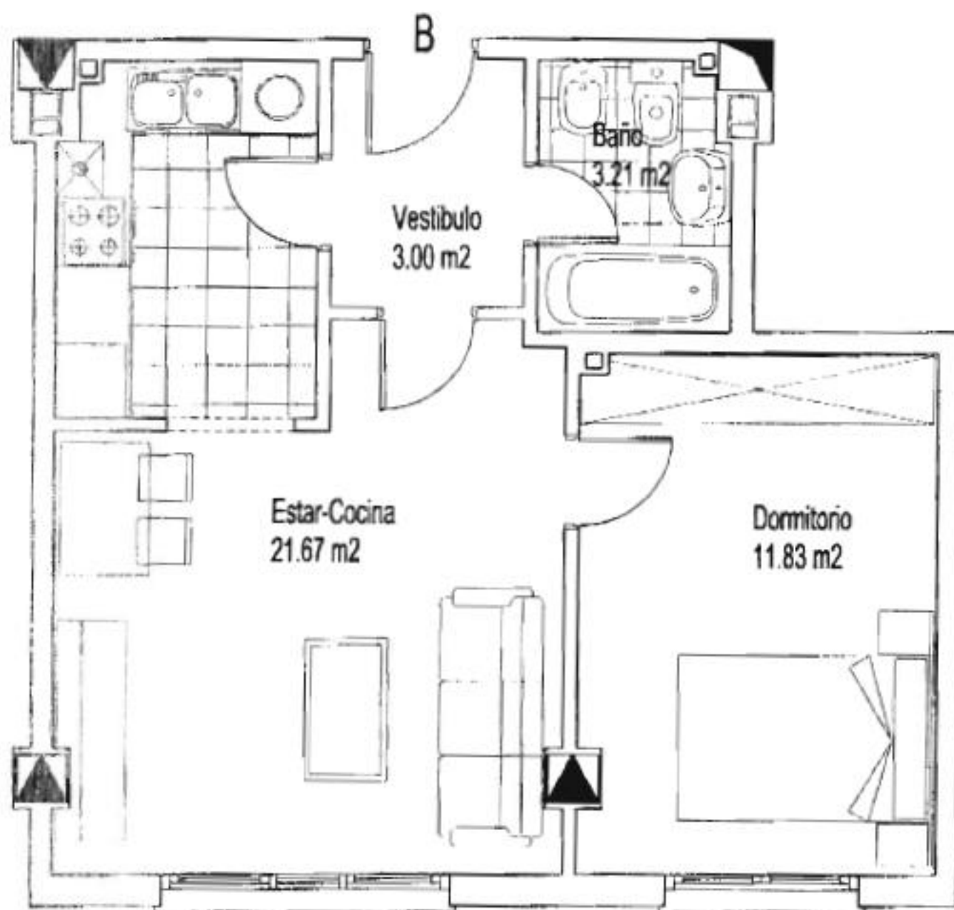
VIVIENDA B PLANTA PRIMERA Y SEGUNDA - MUEBLES BLOQUE 3 ESCALA 1/50
